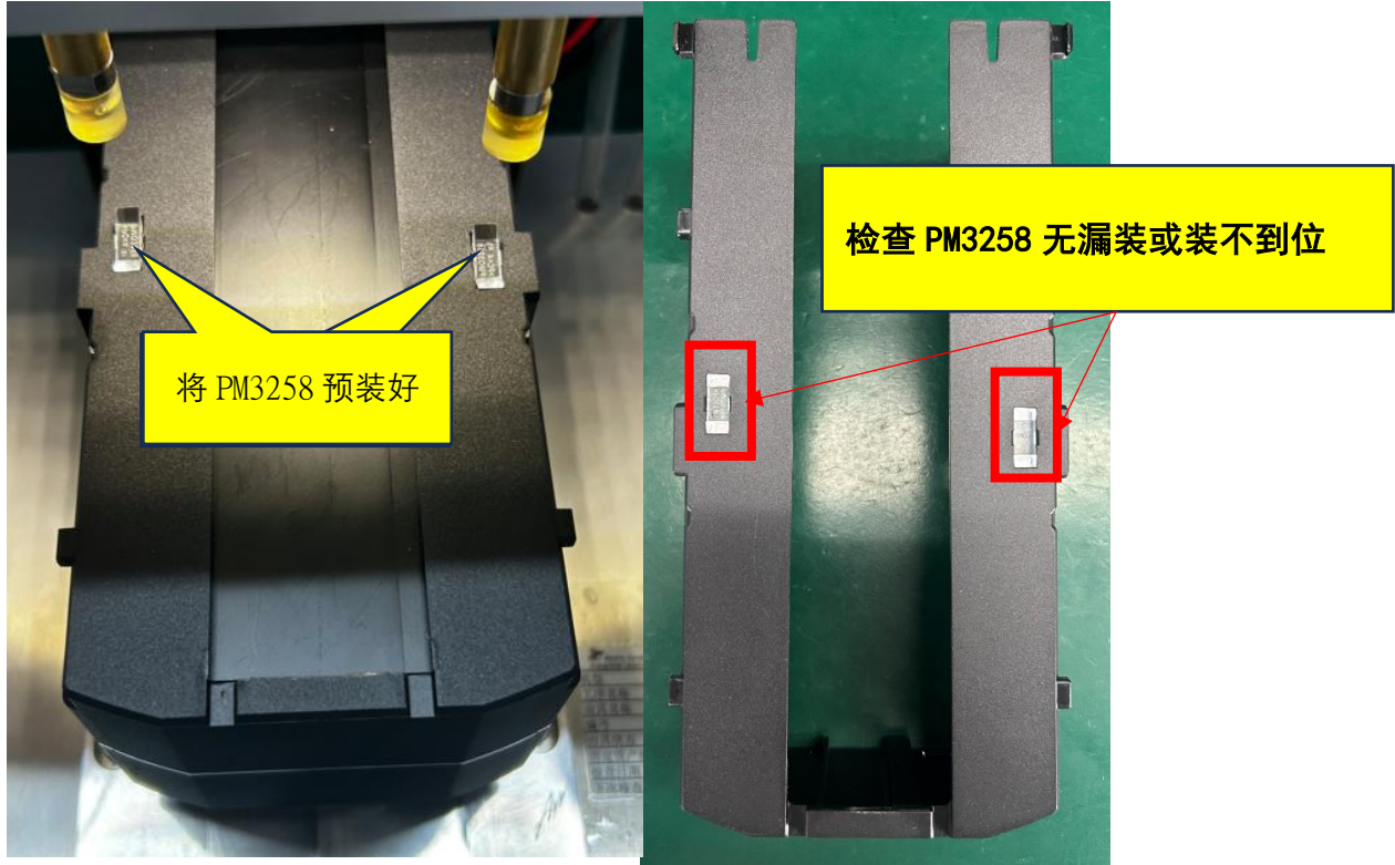
图二，将 PM3085 先放入治具，在将两个 PM3258 预装好，再进行压合，压合到位后取出检查物料无漏装或压合不到位。
